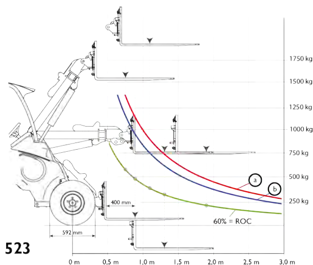
Diagramma di carico - 523/528/530
